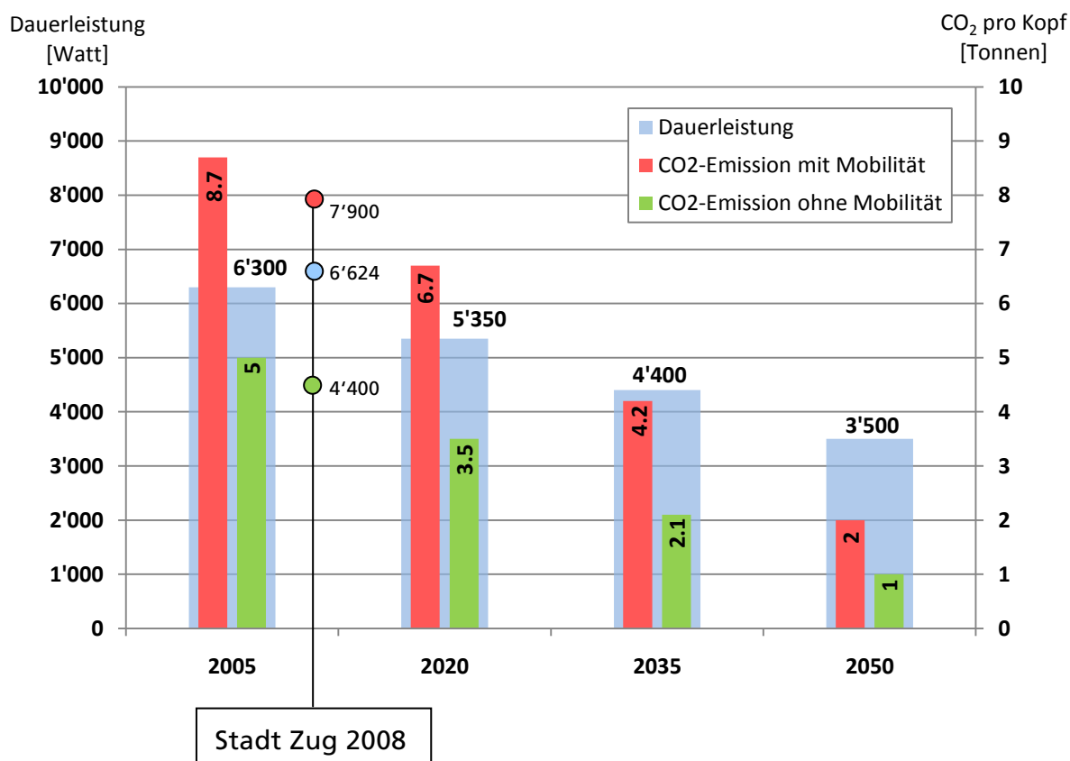
Grafik 2 (absolute CO 2 - und Leistungsziele bis 2050)
