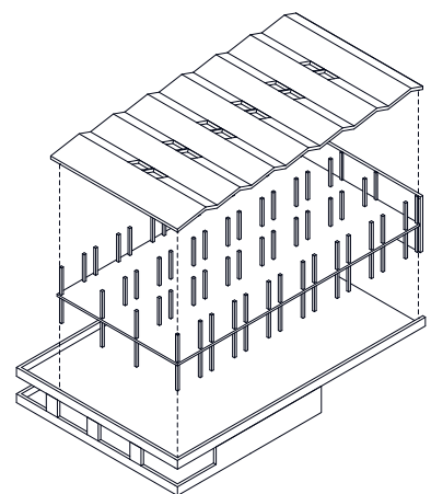
Tragstruktur
