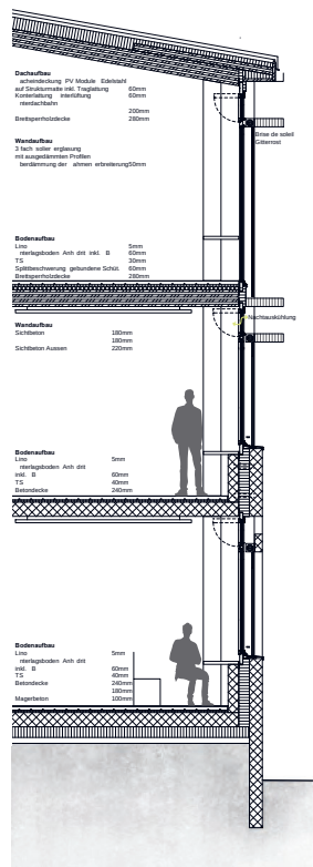
Fassadenschnitt
