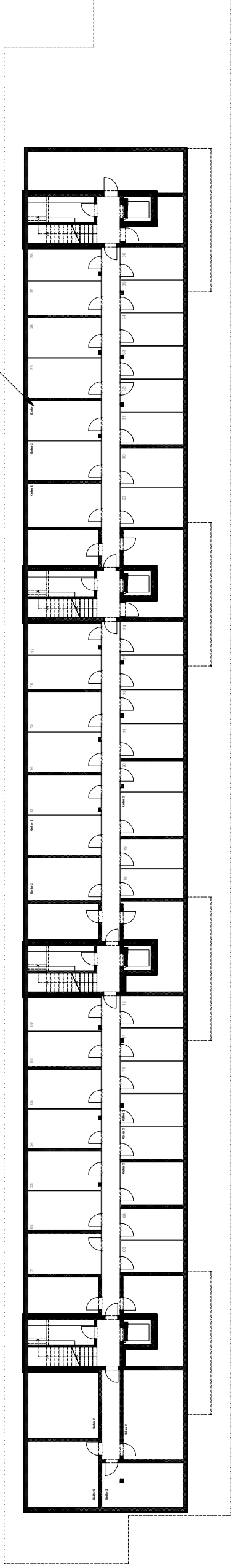
Stand November 2009 Gebäude C _ Untergeschoss
