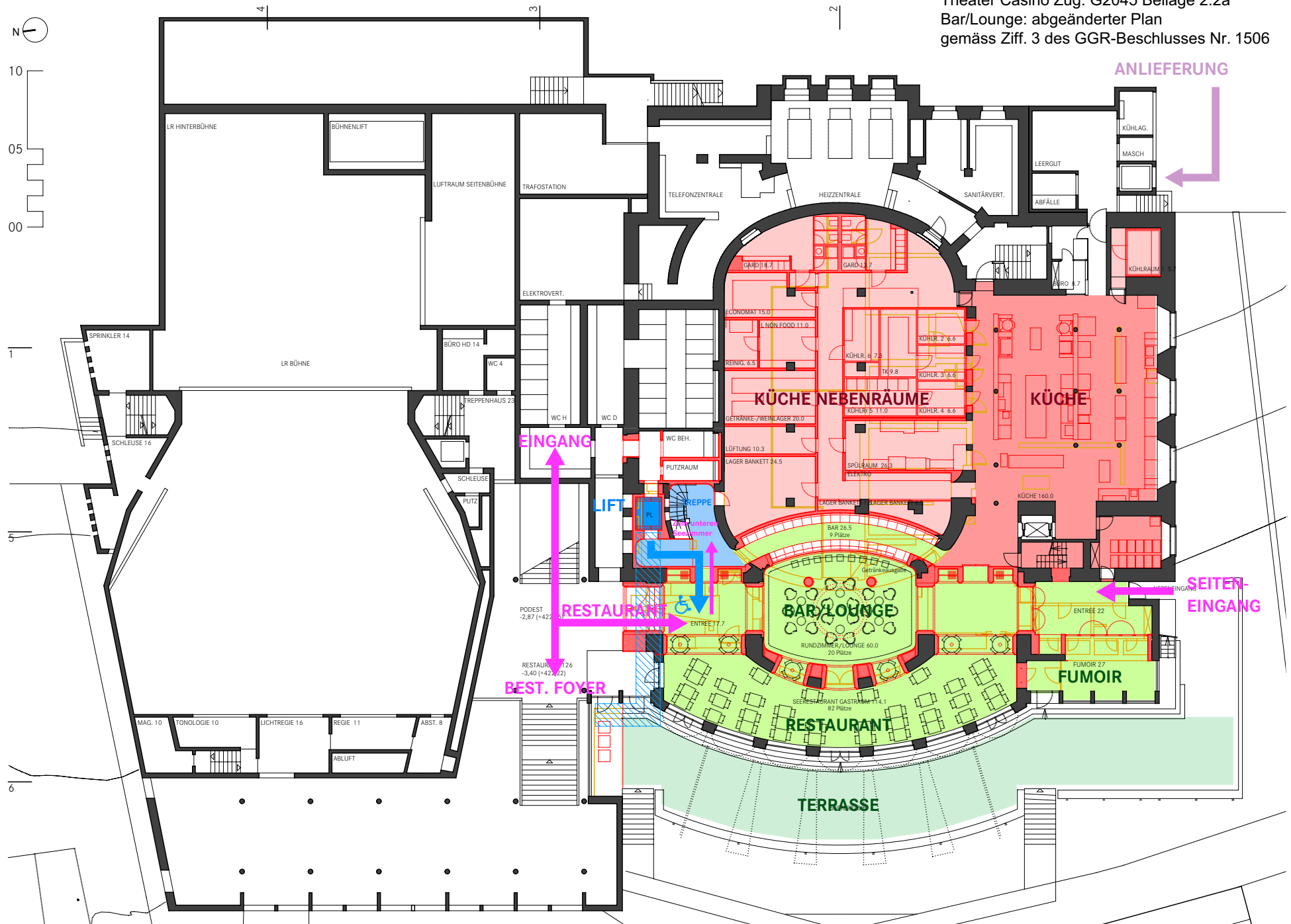
Grundriss Restaurantgeschoss Masstab 1:320
