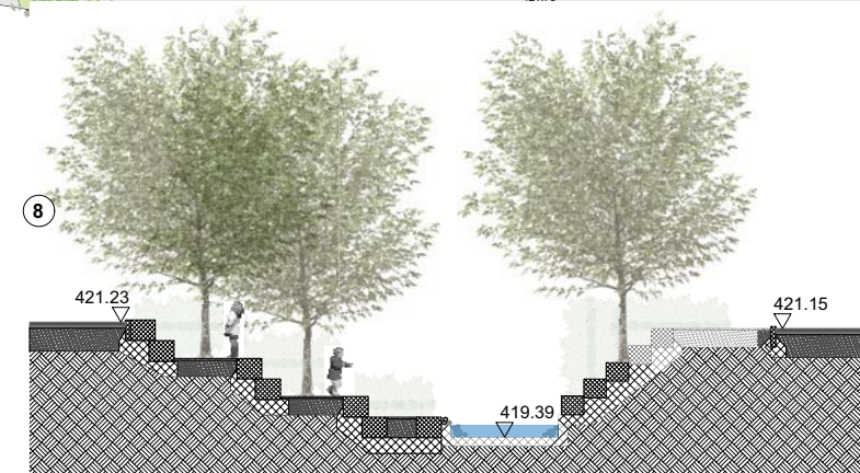
Schnitt A-A' M 1:100
