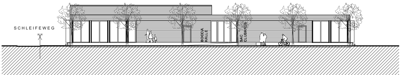
WESTFASSADE
