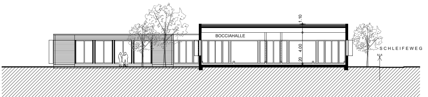
SCHNITT D - D
