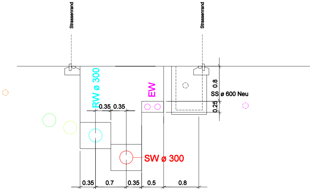
Profil 7
