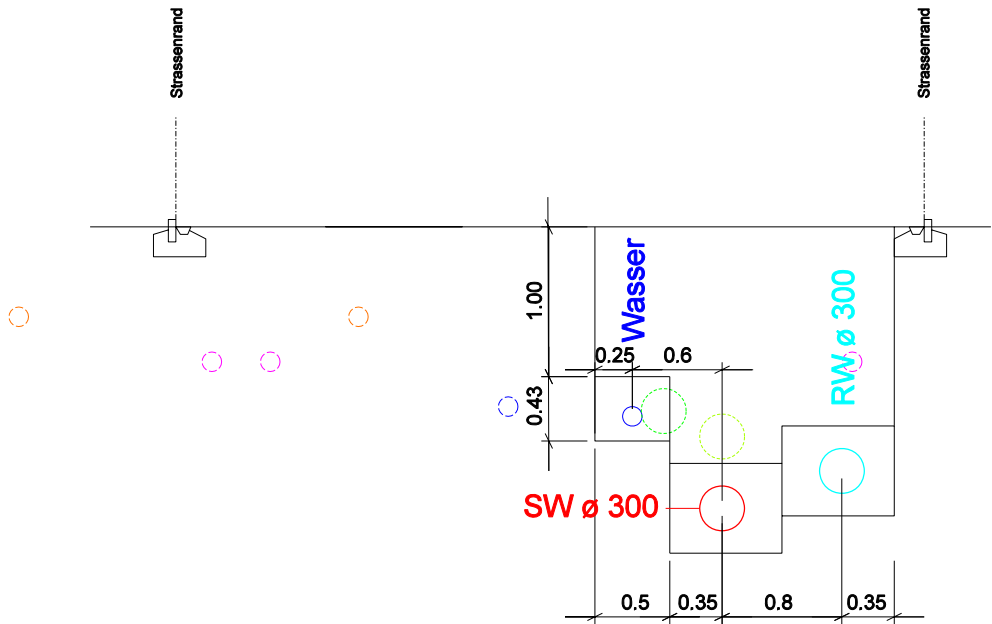
Profil 5
