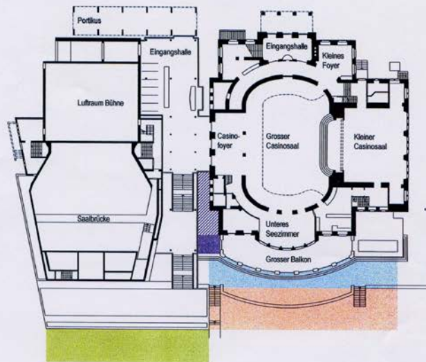
Grundriss Eingangsgeschoss
