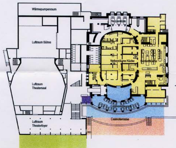
Grundriss Restaurantgeschoss
