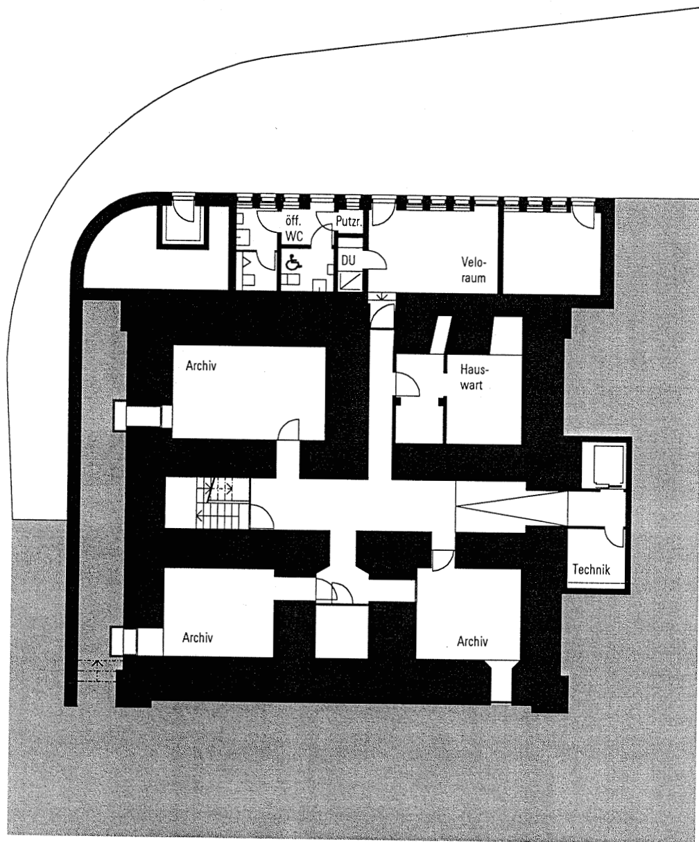
Untergeschoss M: 1:200
