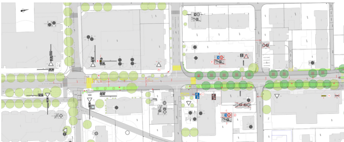
Abbildung 7: Quartier Guthirt (Industriestr. Süd), Abschnitt Süd Situation 1:200, Signalisation + Markierung, Generalplaner IG TZB Zug+, Emch + Berger WSB AG, 13.05.2022
